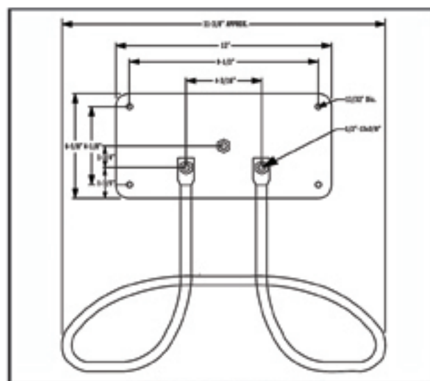
VISTA DELANTERA
